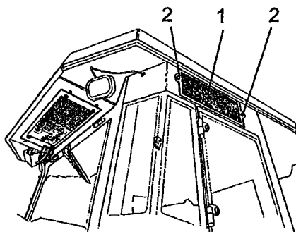
Fig. Cabina 1. Filtro dell'aria pulita 2. Vite (2 pezzi)
