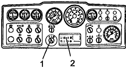
Fig. Quadro strumenti 1. Interruttore di avviamento 2. Quadro delle spie
