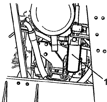
Fig. Vano motore 2. Filtro olio idraulico (x2)
