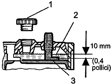
Fig. Livello dell'elettrolito nella batteria
