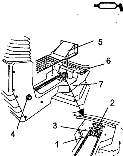
Fig. Supporto del sedile 1. Ingrassatore 2. Ruota dentata 3. Catena dello sterzo 4. Vite di regolazione 5. Coperchio 6. Guide di scorrimento 7. Blocco della rotazione
