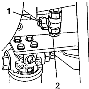
Fig. Lato sottostante del serbatoio idraulico 1. Rubinetto di drenaggio 2. Tappo
