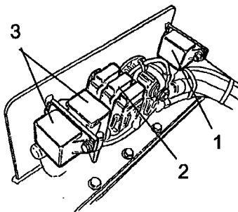
Fig. Vano motore 1. Relè di avviamento 2. Fusibili principali 3. Relè di preriscaldamento
