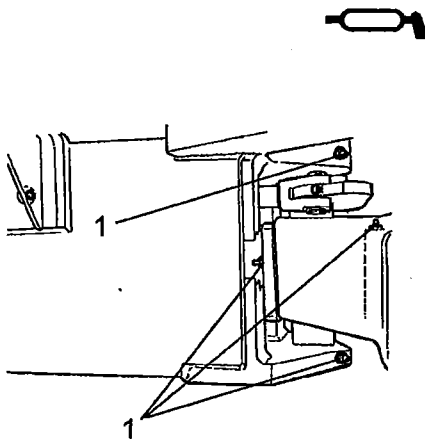
Fig. Snodo, lato destro 1. Ingrassatori, snodo (4 pz)
