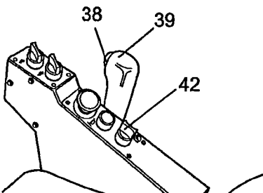
Fig. Quadro di controllo 38. Interruttore delle vibrazioni ON/OFF 39. Leva di comando avanti/indietro 42. Comando del freno di parcheggio
