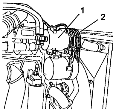
Fig. Vano motore 1. Compressore 2. Cinghia di trasmissione
