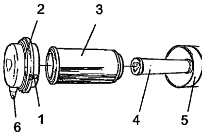
Fig. Depuratore dell'aria
