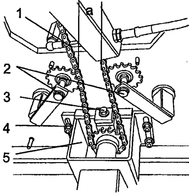
Fig. Sotto la posizione dell'operatore
