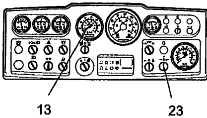
Fig. Quadro strumenti 13. Tachimetro (opzionale) 23. Comando della velocità del motore
