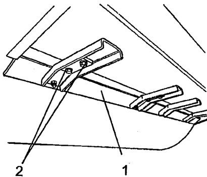
Fig. Raschietti 1. Lame dei raschietti (x4) 2. Viti
