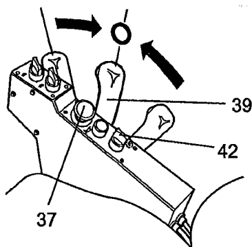
Fig. Quadro di controllo 37. Arresto di emergenza 39. Leva di comando avanti/indietro 42. Comando del freno di parcheggio
