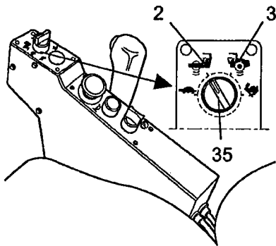
Fig. Quadro di controllo 35. Selettore di velocità, tamburo/ruote (opzionale) 2. Posizione 2 3. Posizione 3
