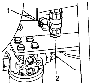
Fig. Lato sottostante del serbatoio idraulico 1. Rubinetto di drenaggio 2. Tappo
