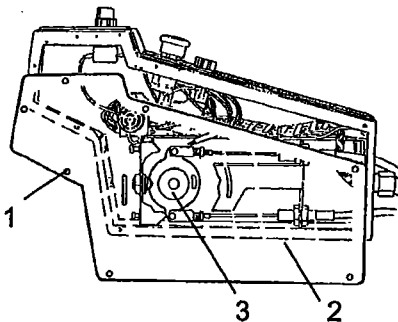
Fig. Leva di marcia avanti/indietro
