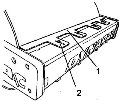
Fig. Raschietti 1. Lame dei raschietti 2. Viti (4)
