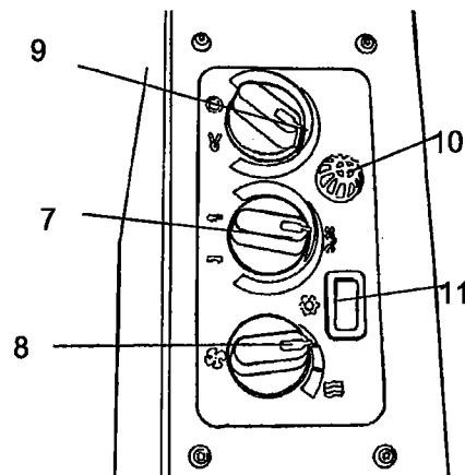
Fig. Lato destro della cabina (aria condizionata opzionale)
