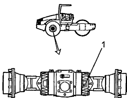
Fig. Controllo del livello nella scatola del differenziale 1. Tappo di livello/riempimento
