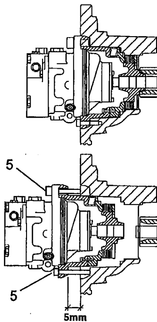
Fig. Freno del tamburo 5. Vite
