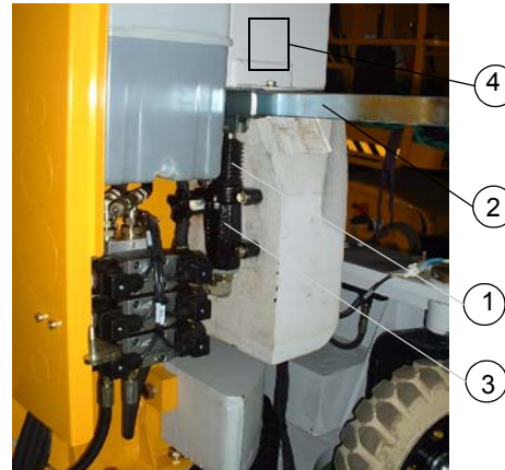
Foto 7 : Pompa a mano
