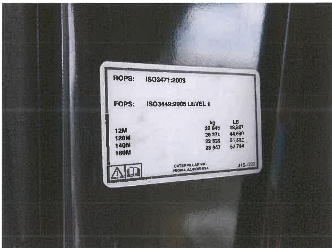
Targa identificativa della struttura protettiva della cabina di guida
