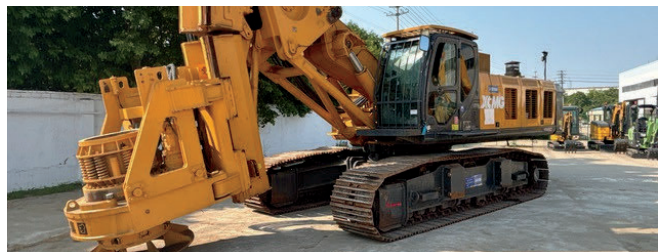
2019 XCMG XR280D
