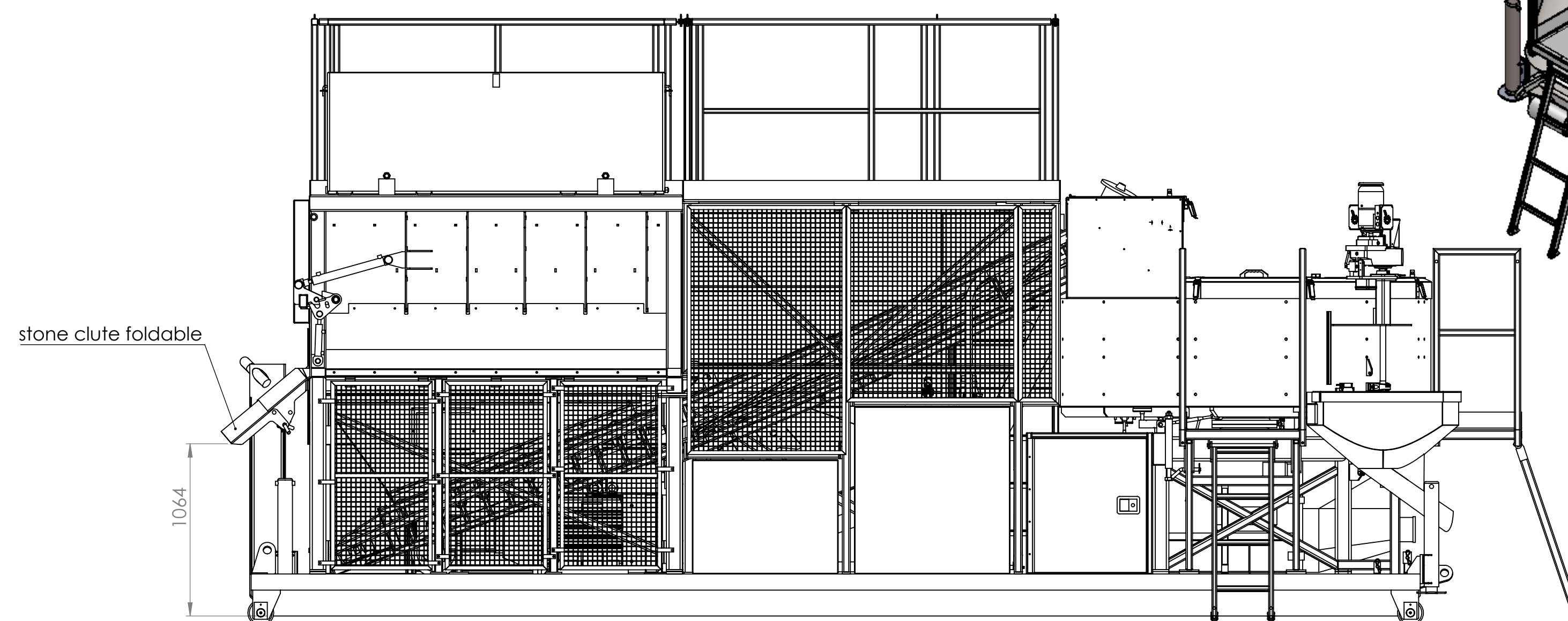
SECTION A-A
