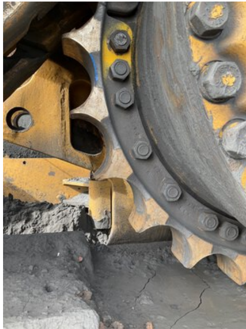
Right Sprockets 1
